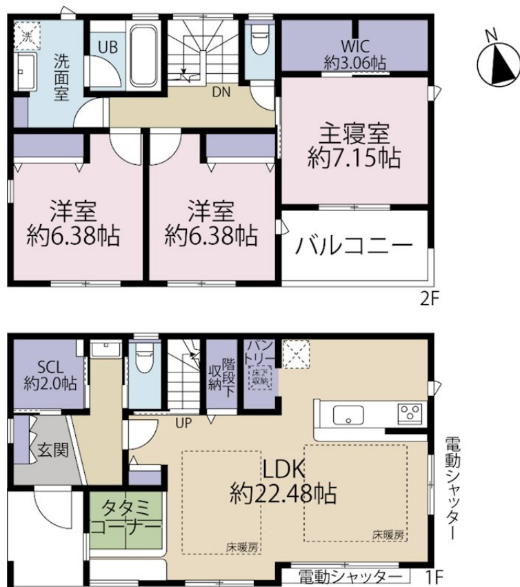
【間取り図】
