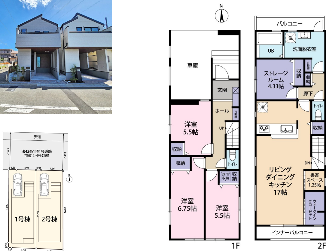
【間取り図】
