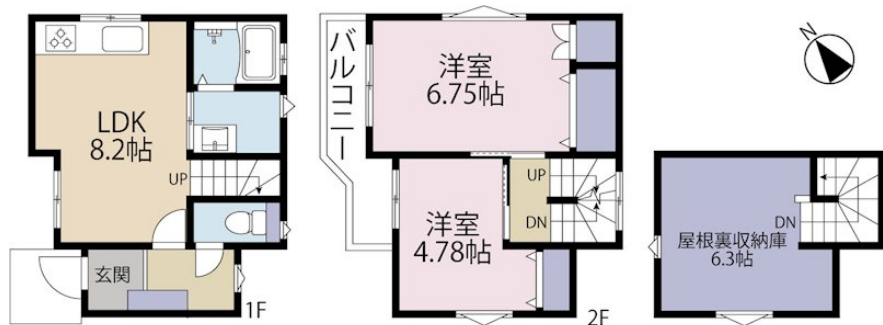
【間取り図】
