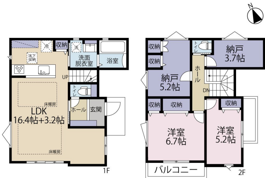
【間取り図】
