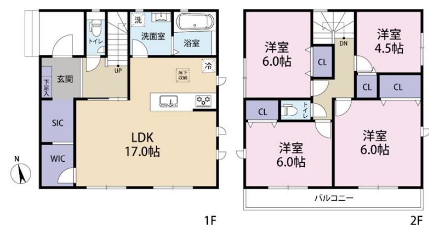
【間取り図】
