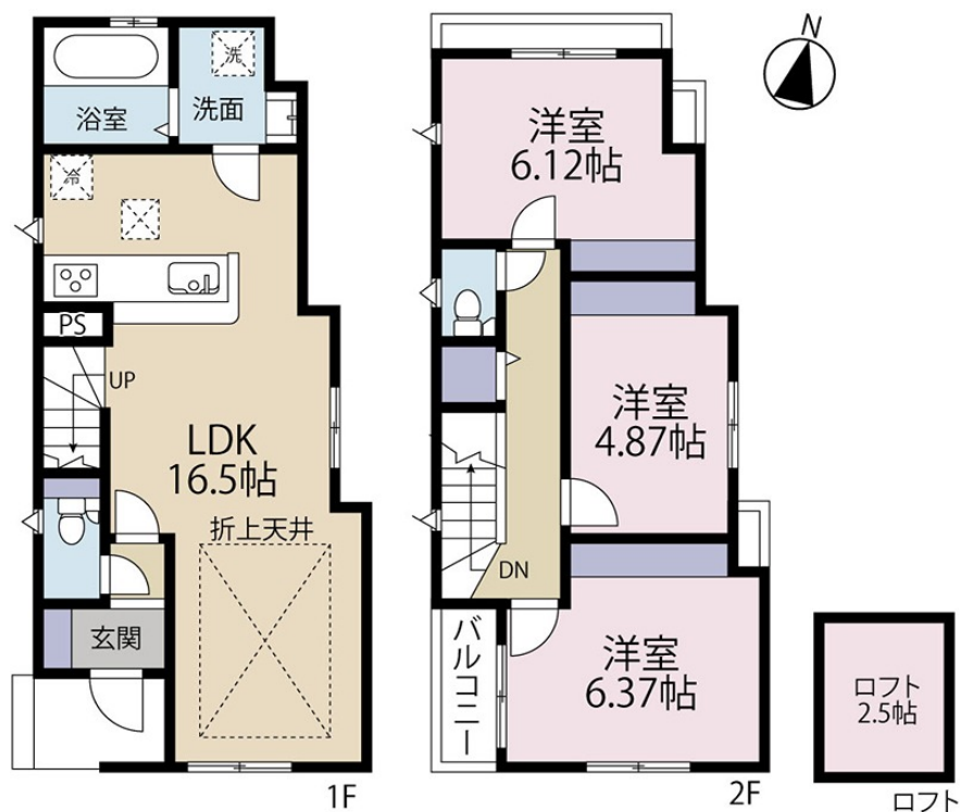
【間取り図】
